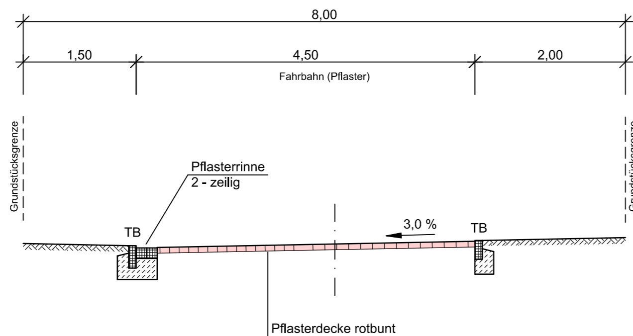
Schnitt Var. 1
