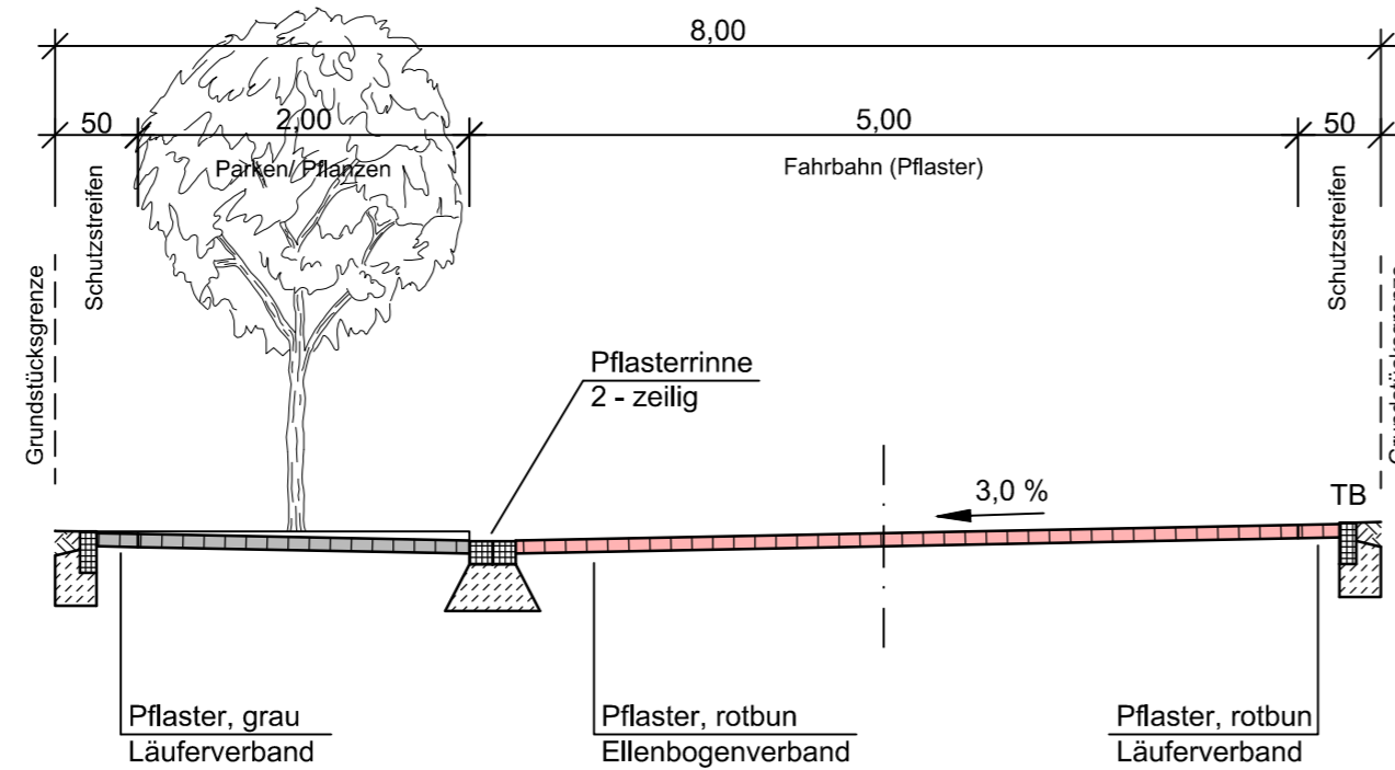
Schnitt Var. 2
